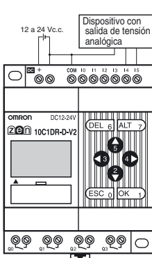
(Modelo con fuente de alimentación de c.c.) Entrada analógica 1: I4 Entrada analógica 2: I5
