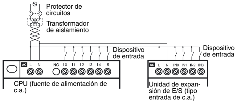
Fuente de alimentación de c.a.
