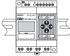
Instalación estándar (vertical)
