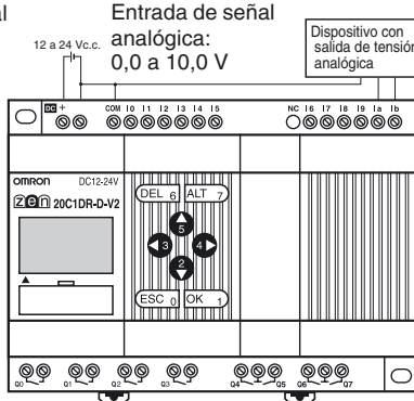
Entrada analógica: la Entrada analógica: lb Modelo con fuente de alimentación de c.c.
