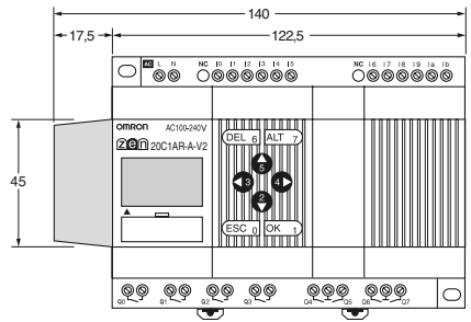
CPU con 20 puntos de E/S
