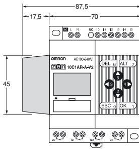
CPU con 10 puntos de E/S
